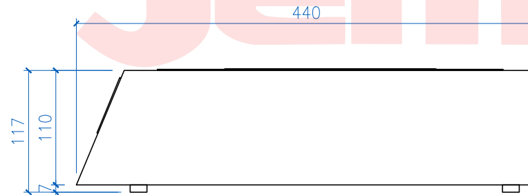
3 IND3500 SIDE Scale:1 : 5
