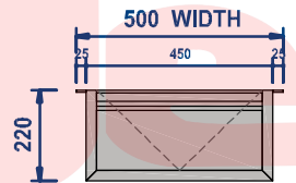
SSDR1 FRONT Scale : 1 : 20M
